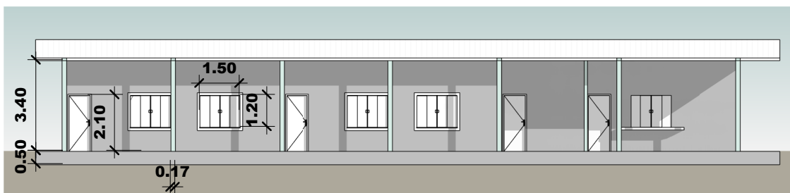
1 CORTE A
