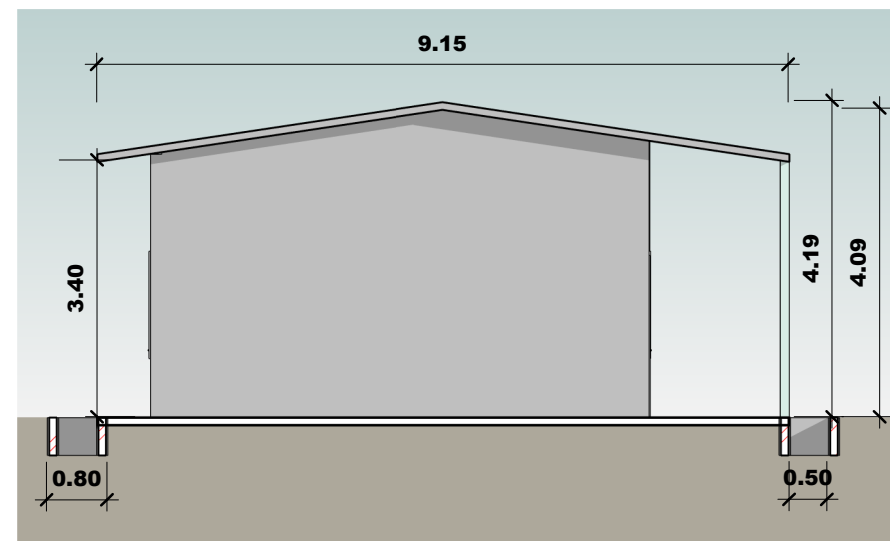
3 CORTE C
