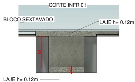
3 CT-01 1 : 15
