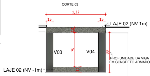
7 CT-03 1 : 15
