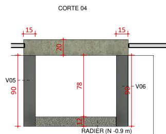
5 CT-04 1 : 15
