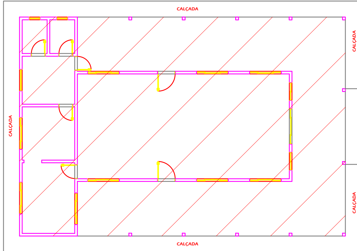
② PLANTA BAIXA - EXISTENTE ESCALA: 1/50
