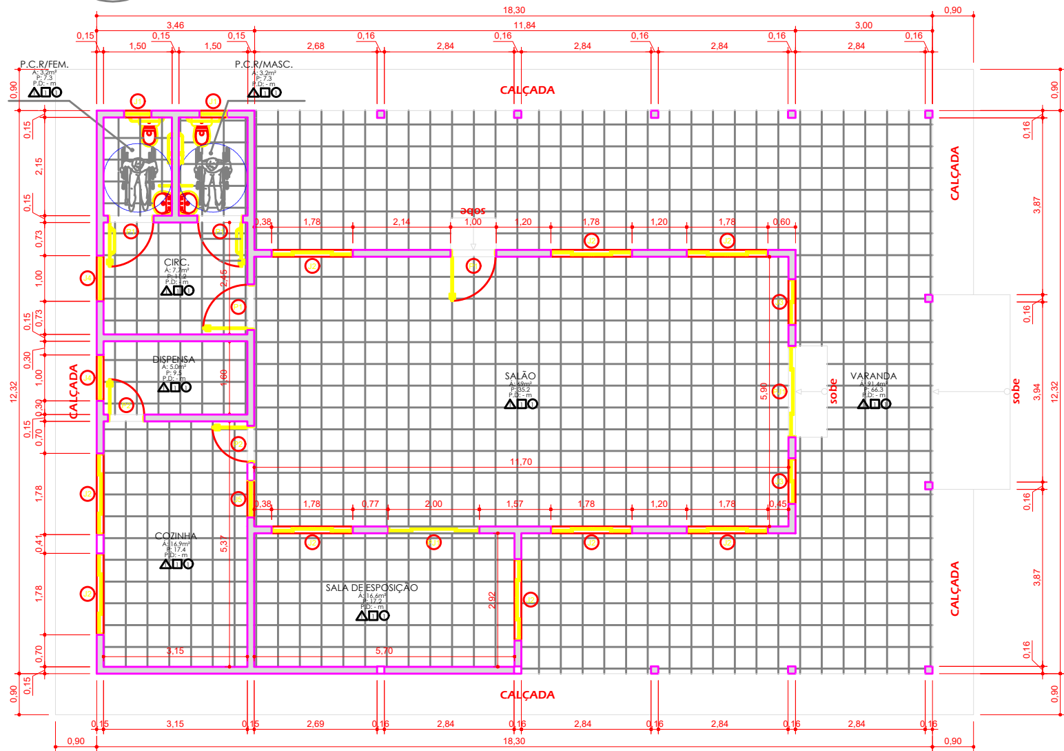
2 PLANTA BAIXA ESCALA: 1/50
