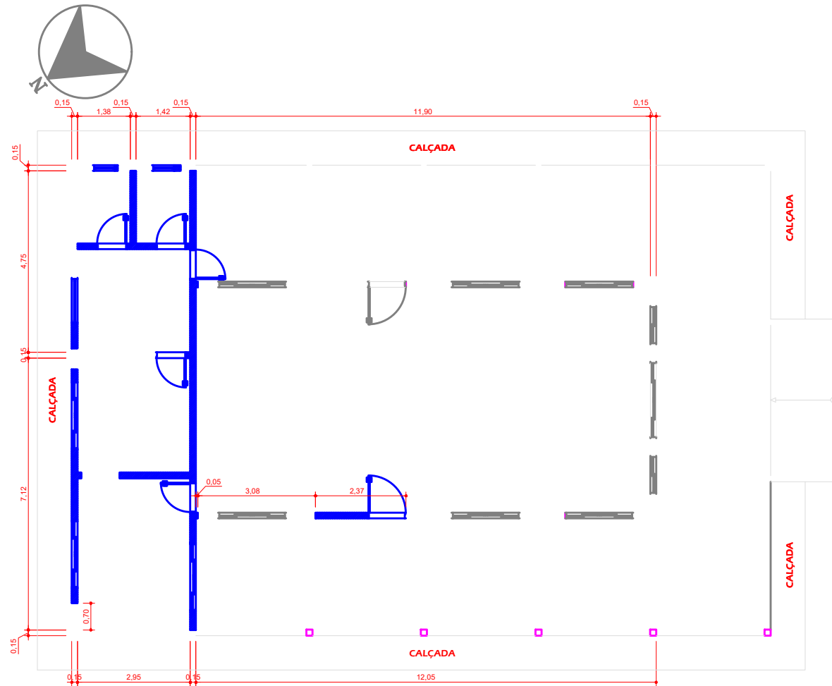
② PLANTA BAIXA - PLANTA A SEREM DEMOLIDAS ESCALA: 1/50
