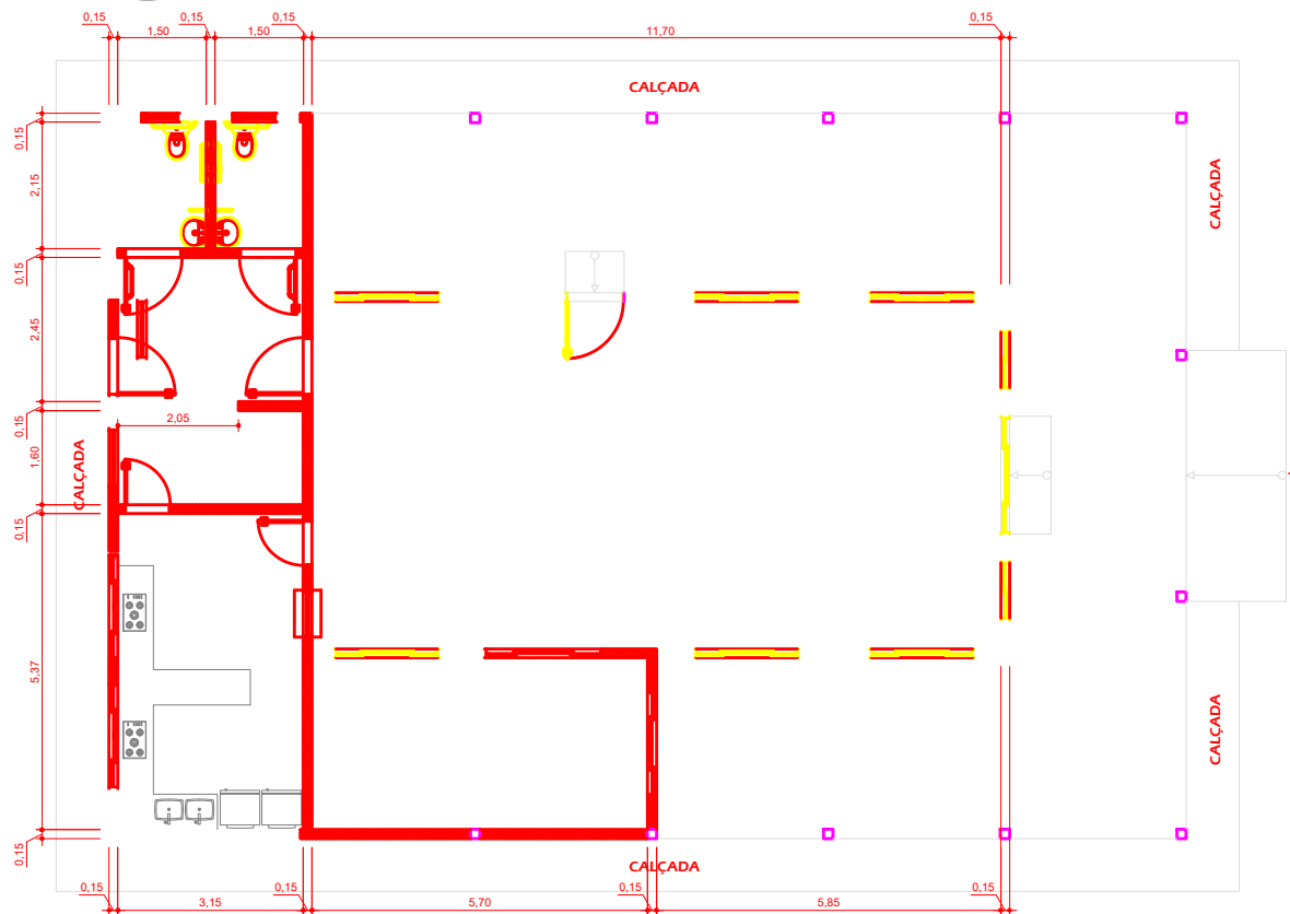
② PLANTA BAIXA - PLANTA A SEREM DEMOLIDAS ESCALA: 1/50
